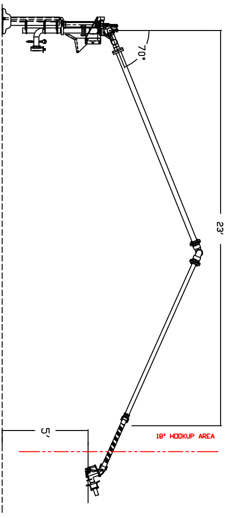
104-HP-2 STRAIT STYLE FUELCRANE
