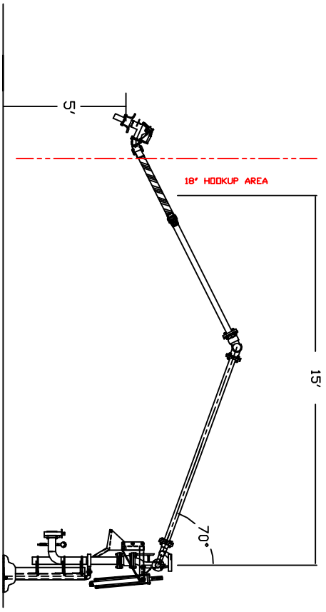
104-HP-1 STRAIT STYLE FUELCRANE
